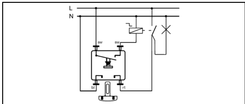
Schakelschema 534 EU
