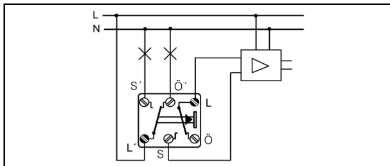
Schakelschema 533-2 U
