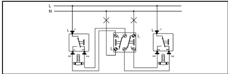
Schakelschema
