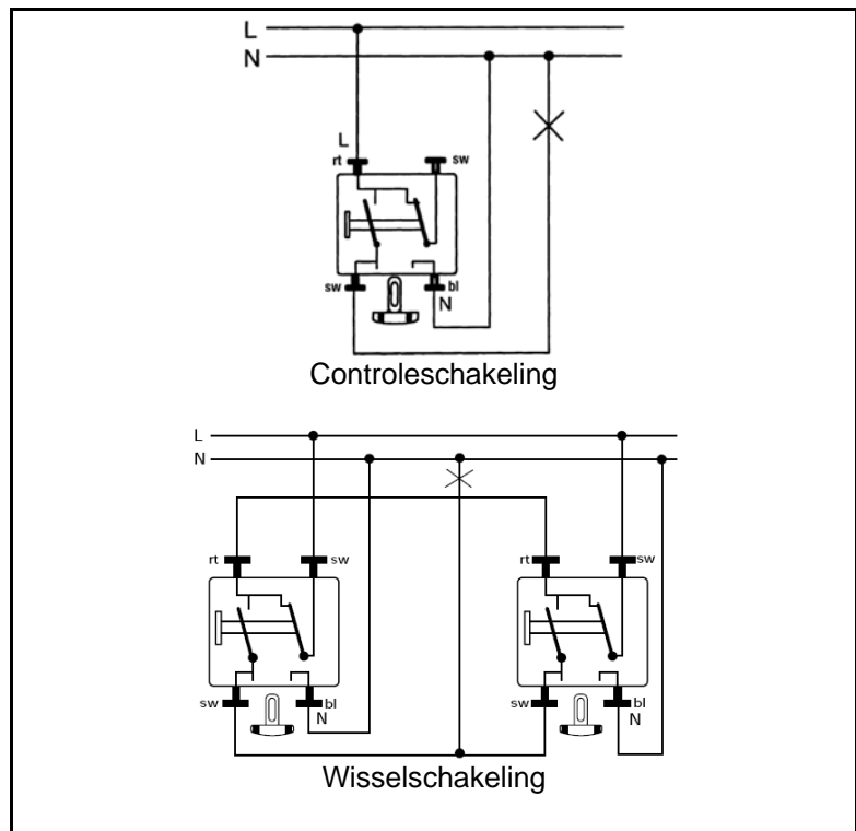
Schakelschema 506 KOETU
