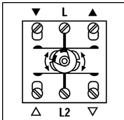
Contact aansluitingen
