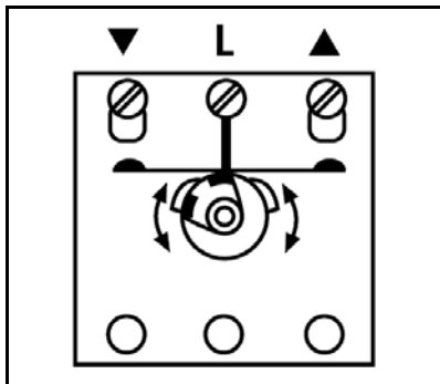
Contact aansluitingen
