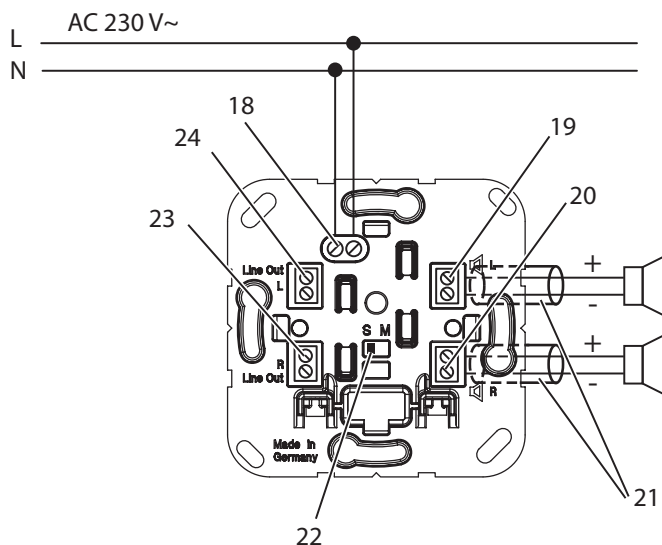
Afb. 4: Aansluiting luidspreker
