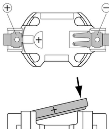
Afbeelding 8: Batterij plaatsen
