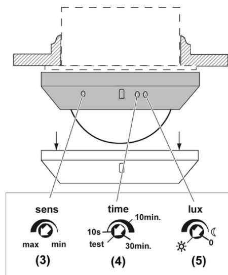
Afbeelding 4: Testinstelling
