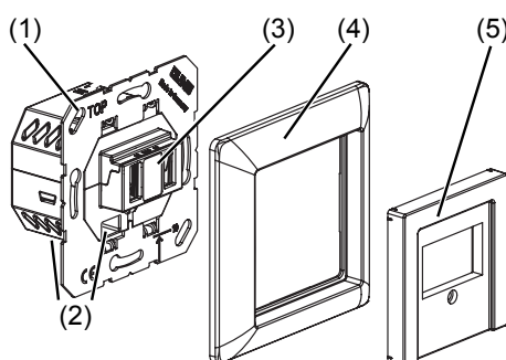
Afb. 1: Constructie apparaat
