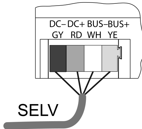
Afbeelding 1: Aansluitschema buskabel
