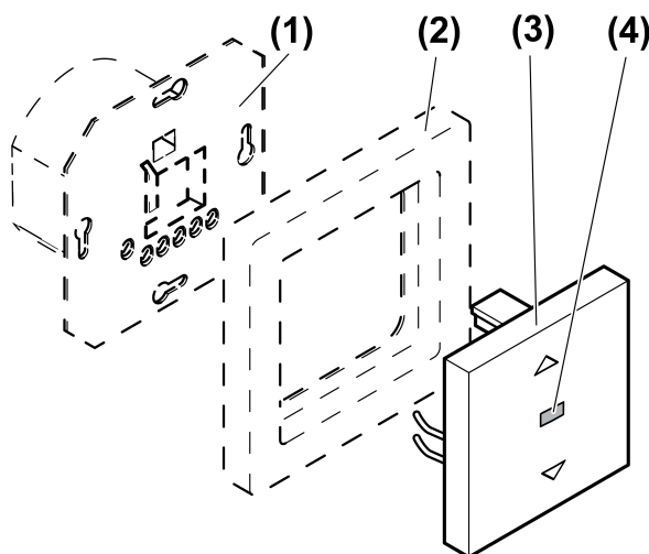
Afbeelding 1: Constructie apparaat
