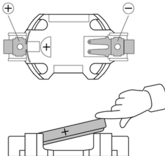
Afbeelding 3: Batterij plaatsen
