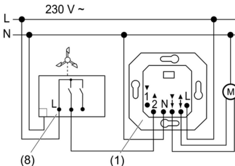
Afbeelding 5: Aansluitvoorbeeld windsensor
