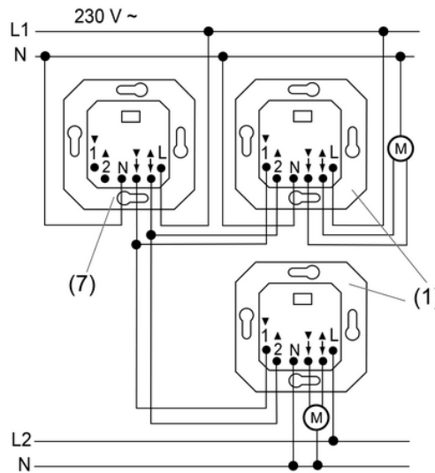
Afbeelding 3: Aansluitvoorbeeld groepsbesturing
