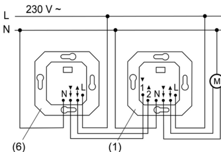
Afbeelding 2: Element met nevenaansluiting
