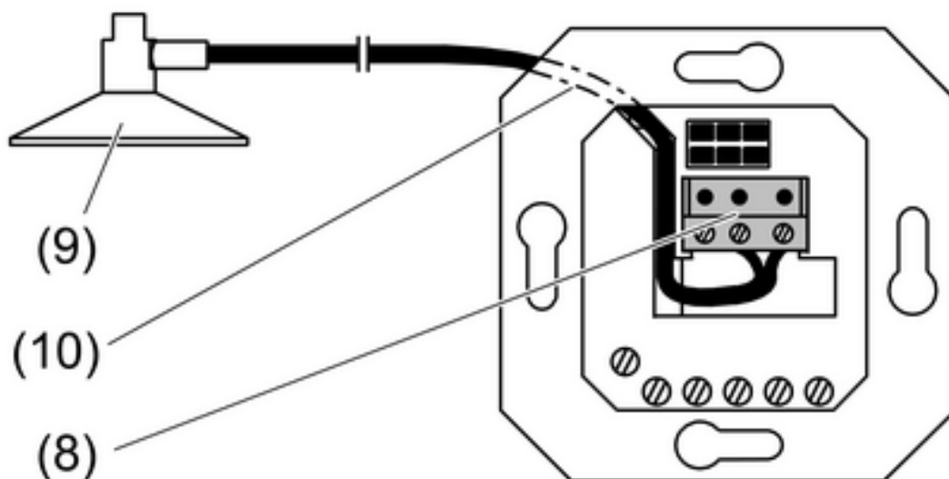
Afbeelding 5: Opbouwinstallatie sensorkabel
