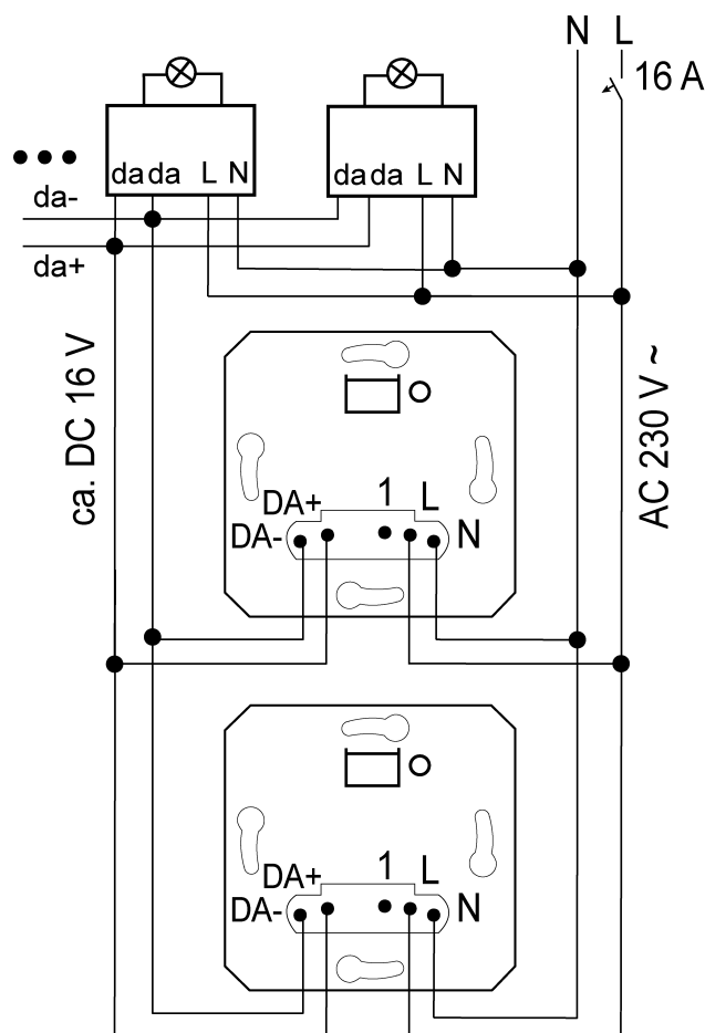
Afbeelding 3: Parallel schakelen van DALI-eenheden
