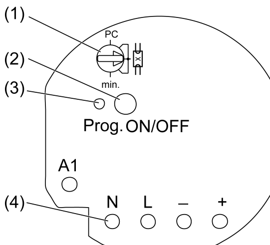
Figura 1: Struttura dell'apparecchio
