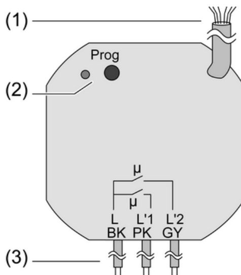
Figure 2: Actionneur de commutation 2 postes
