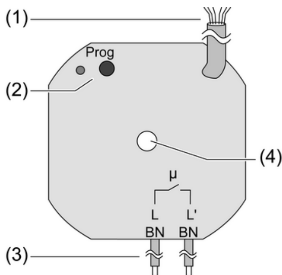
Figure 1: Actionneur de commutation 1 poste
