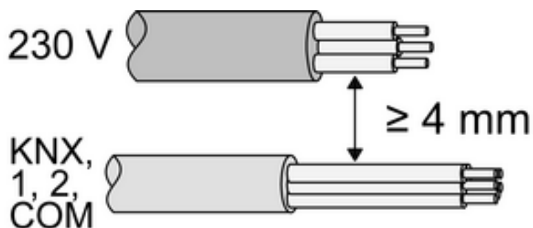
Figure 5: Distance entre le câble secteur et le câble de commande
