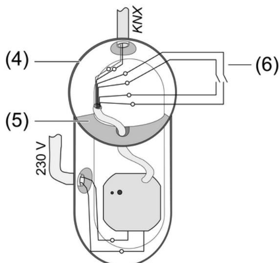
Figure 4: Montage dans un boîtier d'appareillage
