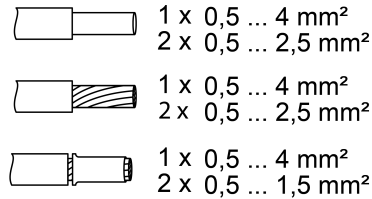
Figure 2: Section de conducteur serrable
