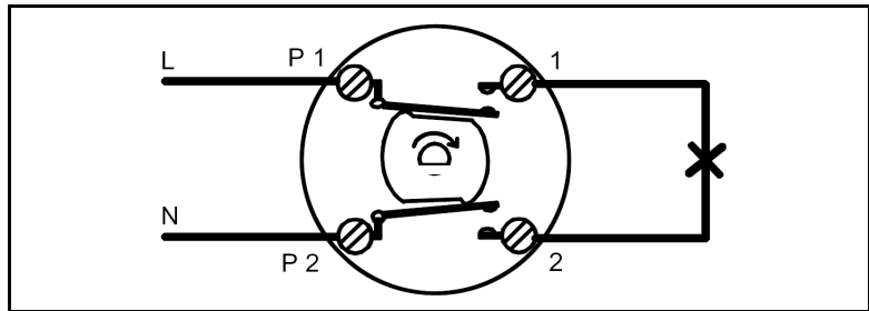
Schémas de raccordement
