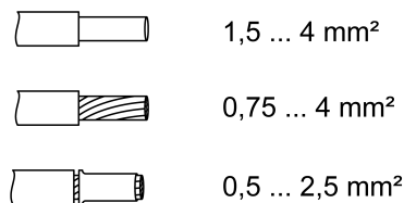
Imagen 3: Sección transversal enchufable del conductor
