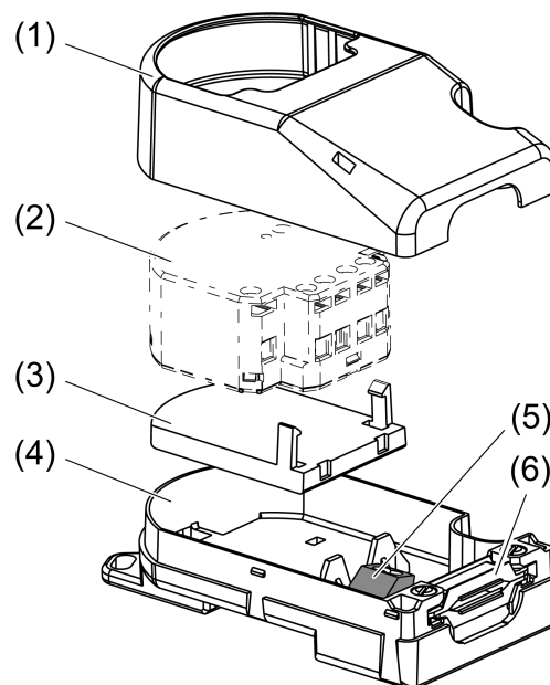
Imagen 1: Componentes de la caja de montaje con aparato eNet
