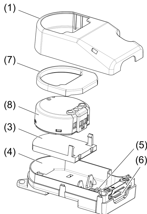
Imagen 2: Componentes de la caja de montaje con regulador de intensidad de luz Mini
