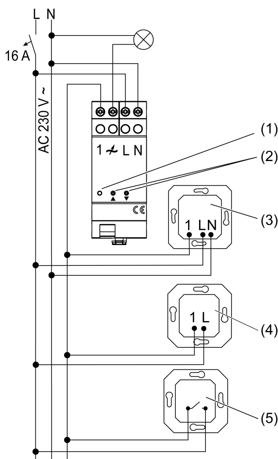
Imagen 1: Plano de conexión
