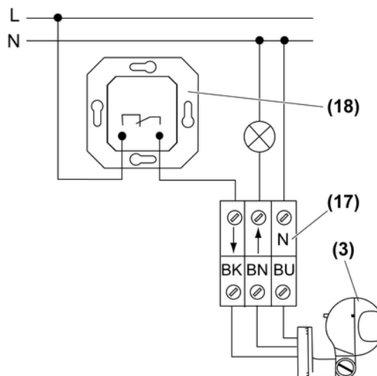
Imagen 8: Diagrama de conexiones
