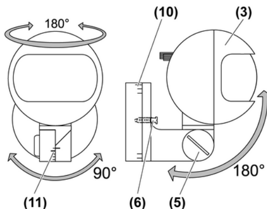
Imagen 3: Orientación del cabezal sensor
