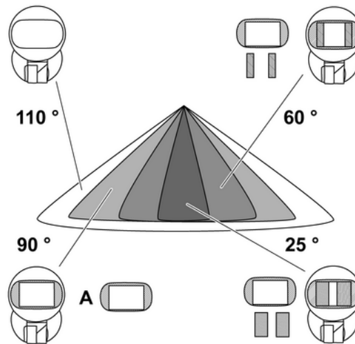
Imagen 4: Área de detección con obturador A.
