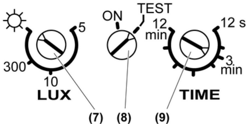
Imagen 2: Regulador
