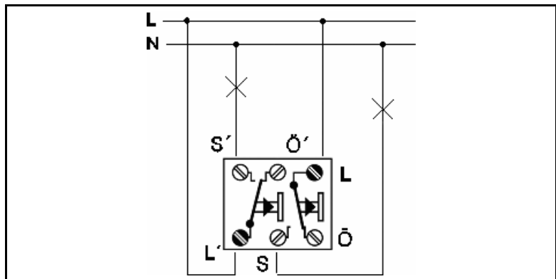
Ejemplos de conexionado 539 U
