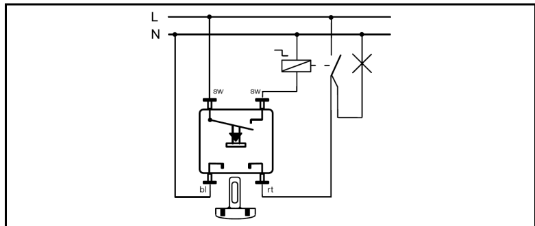
Wiring diagrams 534 U
