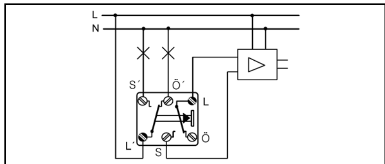
Wiring diagrams 533-2 U
