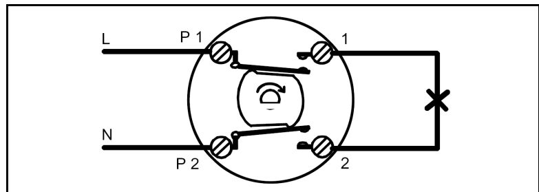
Wiring diagrams
