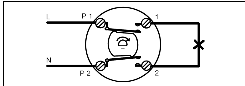
Wiring diagrams
