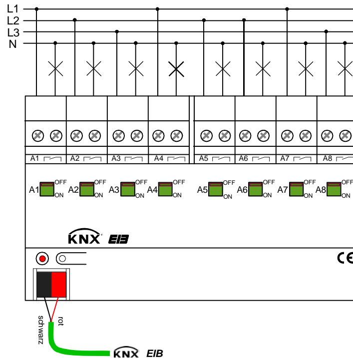
Bild 1: Elektrischer Anschluss
