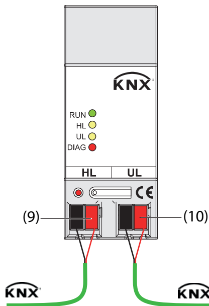
Bild 2: Anschlussplan
