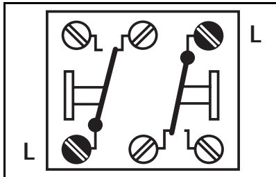
Anschlussklemmen
