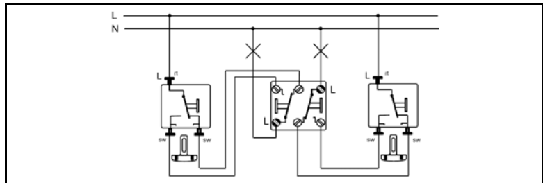
Anschlussbeispiel
