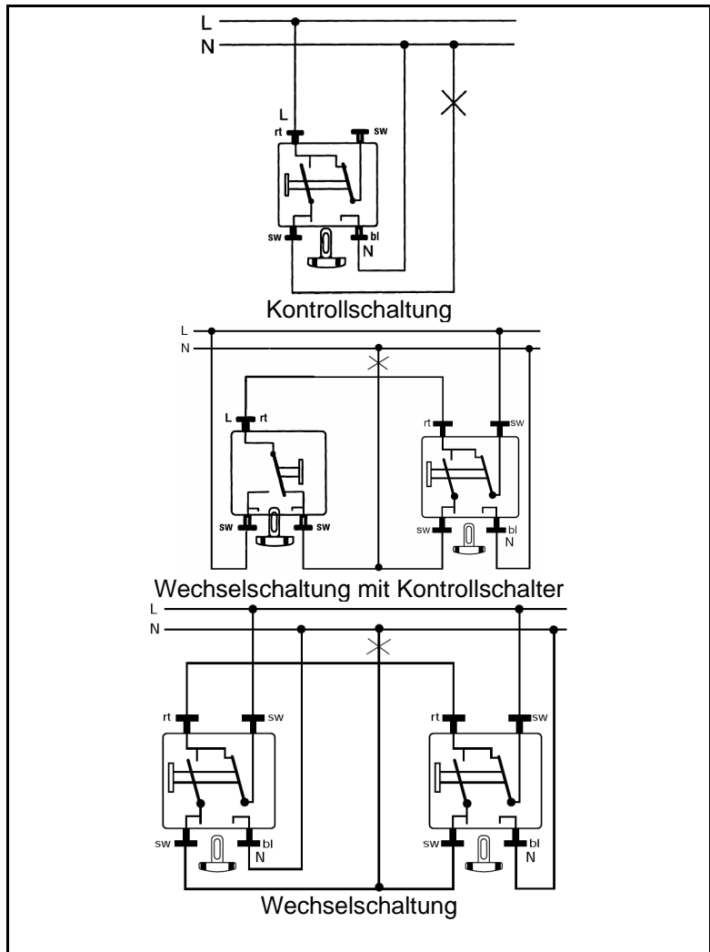
Anschlussbeispiel 506 KOU
