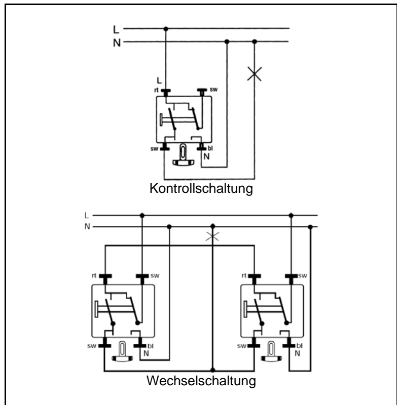
Anschlussbeispiel 506 KOTU
