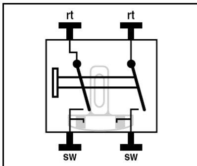
Anschlussklemmen
