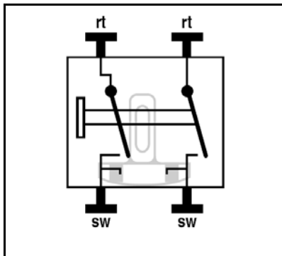
Anschlussklemmen
