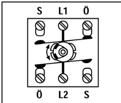
Anschlussklemmen
