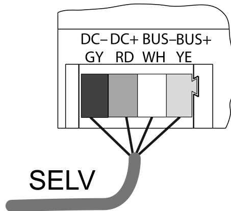
Bild 1: Anschlussplan Busleitung
