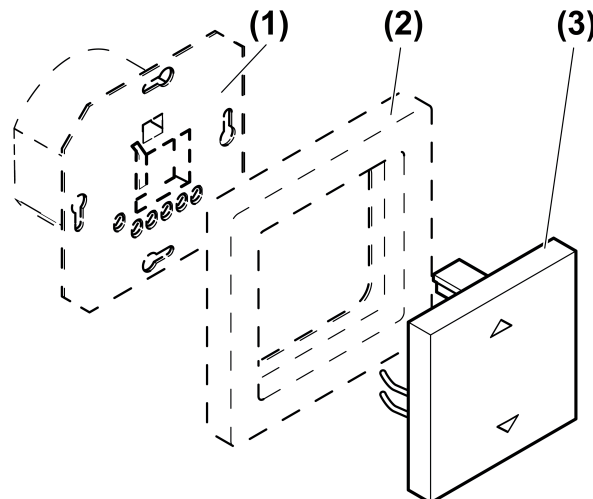
Bild 1: Geräteaufbau
