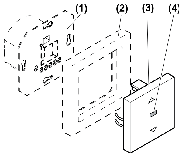
Bild 1: Geräteaufbau
