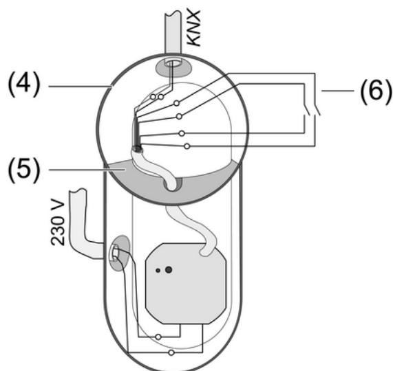
Bild 4: Montage in Gerätedose
