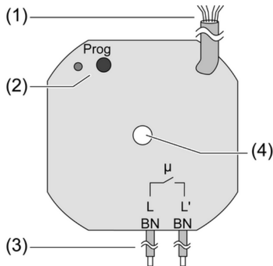
Bild 1: Schaltaktor 1fach
