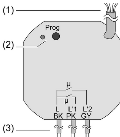
Bild 2: Schaltaktor 2fach
