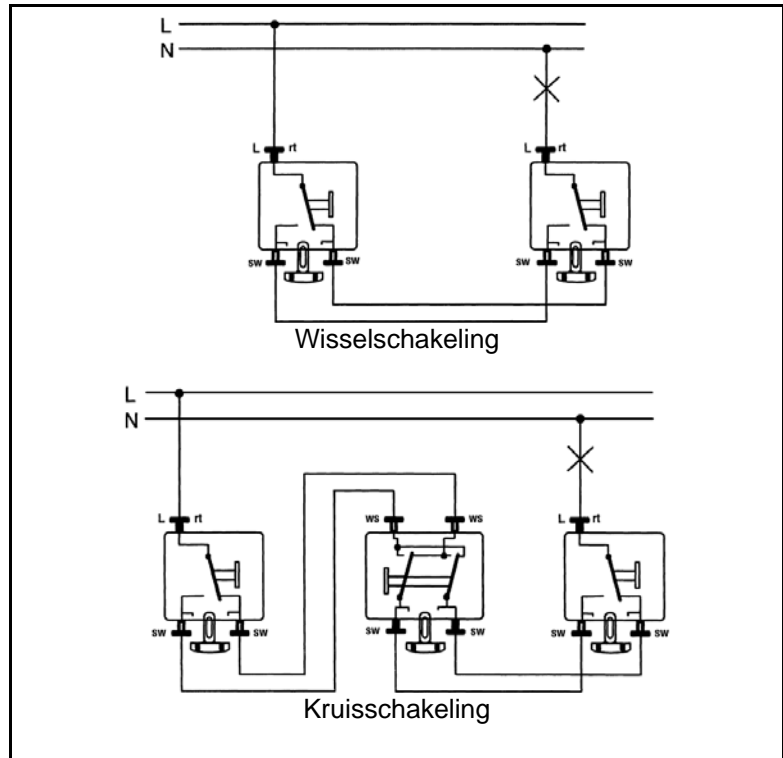
Schakelschema 606 A
