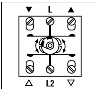
Contact aansluitingen
