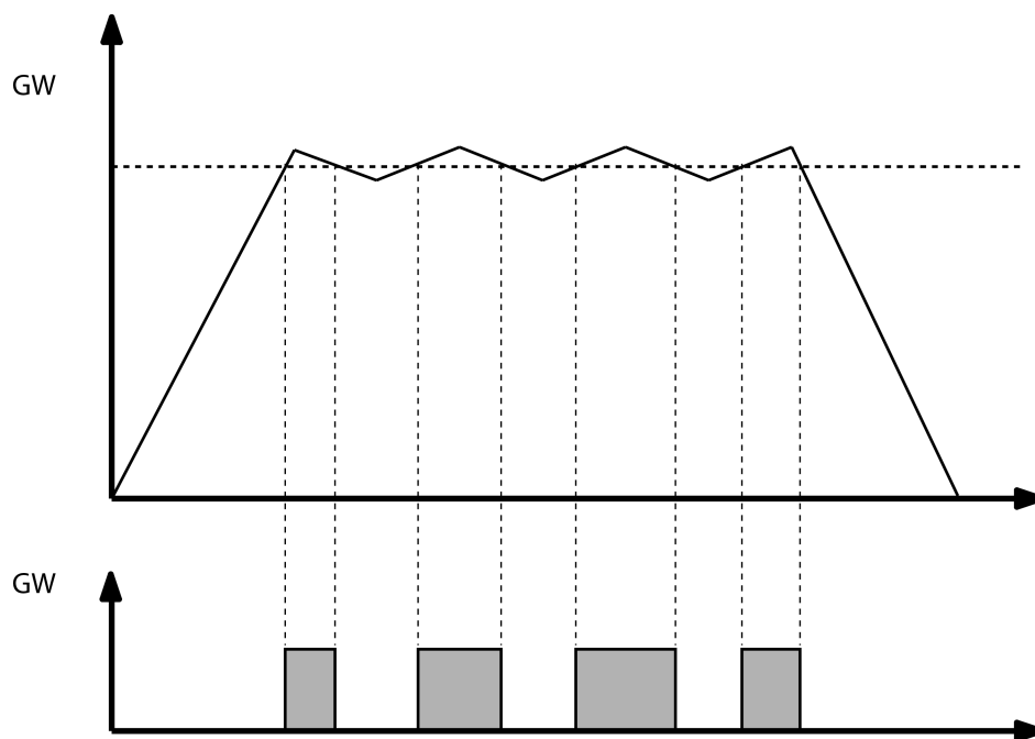
Bild 13: Schalthäufigkeit ohne Hysterese
