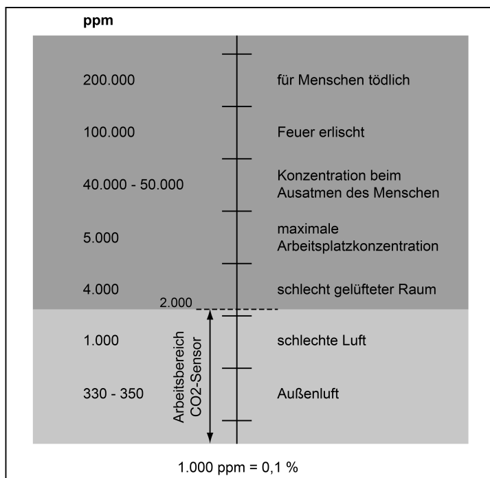
Bild 7: CO 2 -Konzentration
