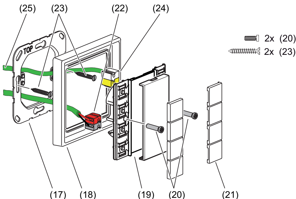
Bild 7: Montage des Tastsensor-Moduls mit Anschluss eines Tastsensor-Erweiterungsmoduls
