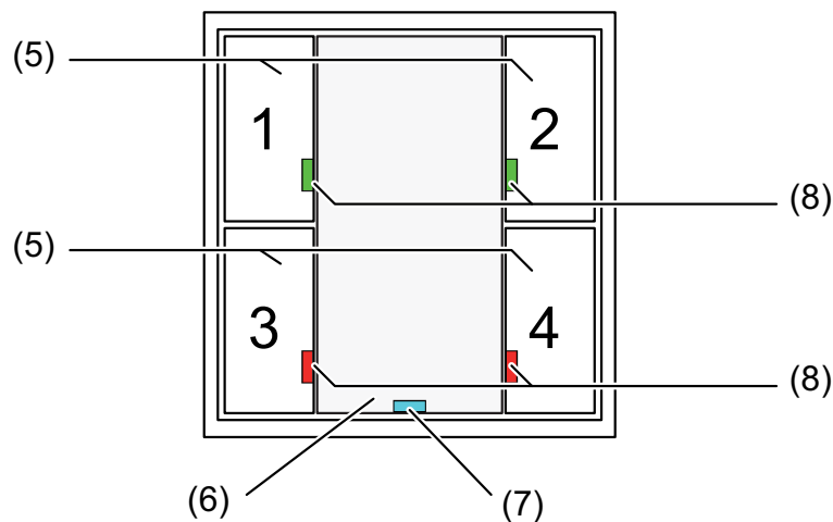
Bild 2: Frontansicht Tastsensormodul Universal 2fach
