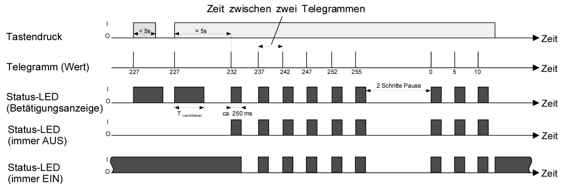
Bild 14: Beispiel zur Wertverstellung mit Wertbereichs-Überlauf
