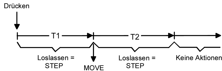
Bild 12: Bedienkonzept "Lang – Kurz oder Kurz"
