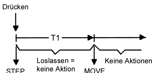
Bild 11: Bedienkonzept "Kurz - Lang"
