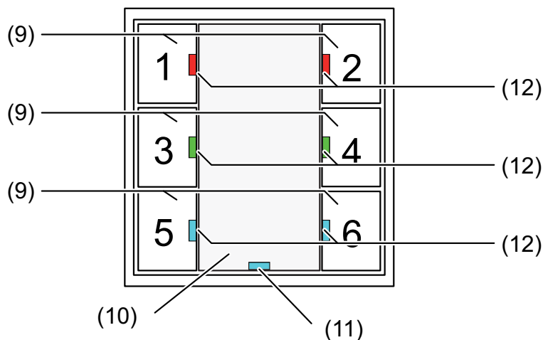
Bild 3: Frontansicht Tastsensormodul Universal 3fach
