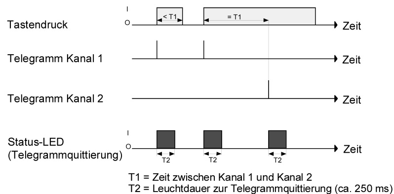
Bild 16: Beispiel zum Bedienkonzept "Kanal 1 oder Kanal 2"
