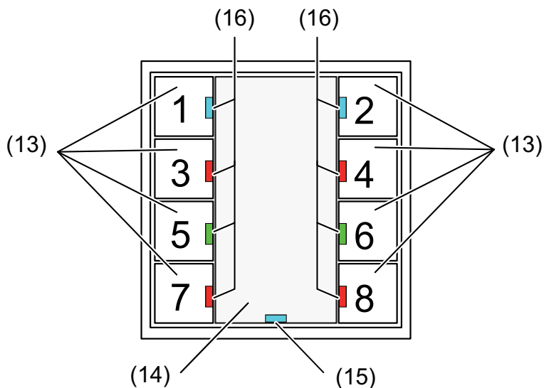
Bild 4: Frontansicht Tastsensormodul Universal 4fach
