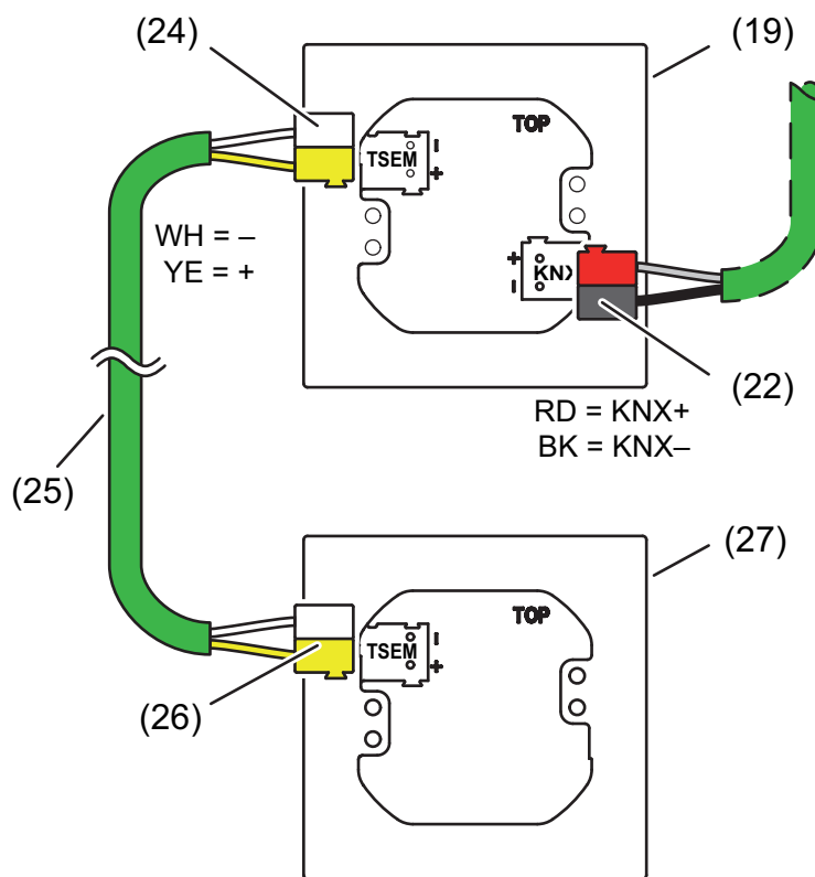
Bild 6: Anschluss des Tastsensor-Erweiterungsmoduls (Ansicht von hinten)
