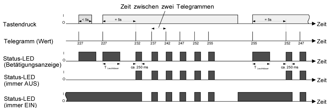
Bild 13: Beispiel zur Wertverstellung ohne Wertbereichs-Überlauf
