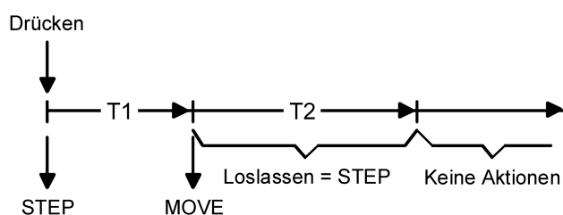
Bild 9: Bedienkonzept "Kurz-Lang-Kurz"
