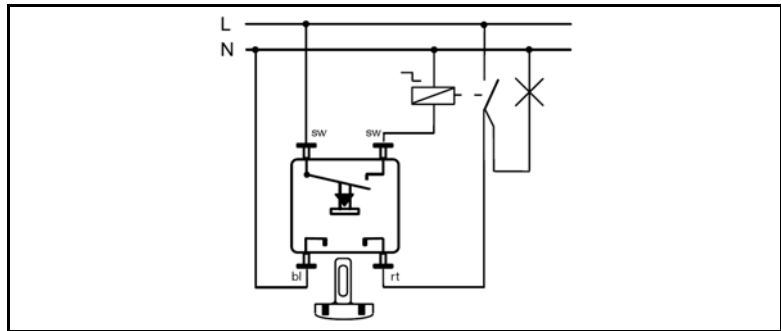
Anschlussbeispiel 834 W
