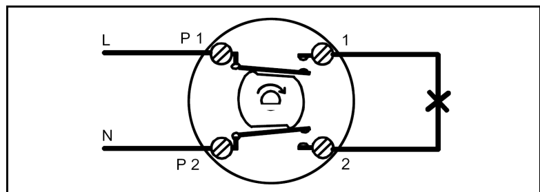
Schaltbild
