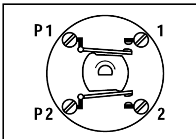
Anschlussklemmen
