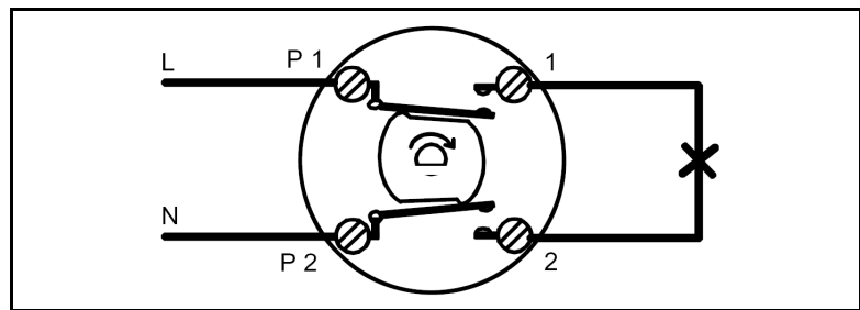
Schaltbild
