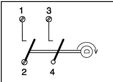
Anschlussklemmen
